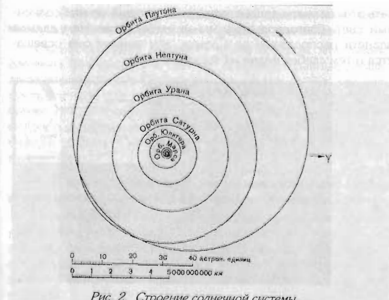
Рис. 2. Строение солнечной системы.
