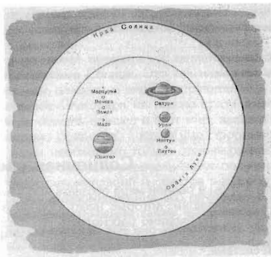
Рис. 1. Сравнительные размеры Солнца и других планет.
