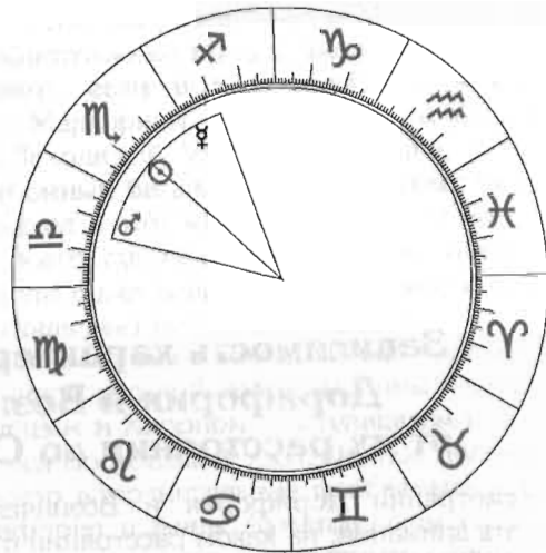
Рис. 10. Расположение Дорифория и Возничего на расстоянии до 28°.
